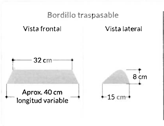
Ilustración 1. Figura 5-6. Dimensiones bordillo traspasable.
