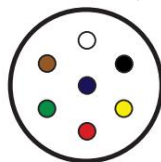
FONDO VIVO DE 7 CABLES (Configuración Gincor)
