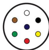
ENCHUFE ISO PRINCIPAL DE 7 CABLES CON VIVO EN LA PARTE INFERIOR
